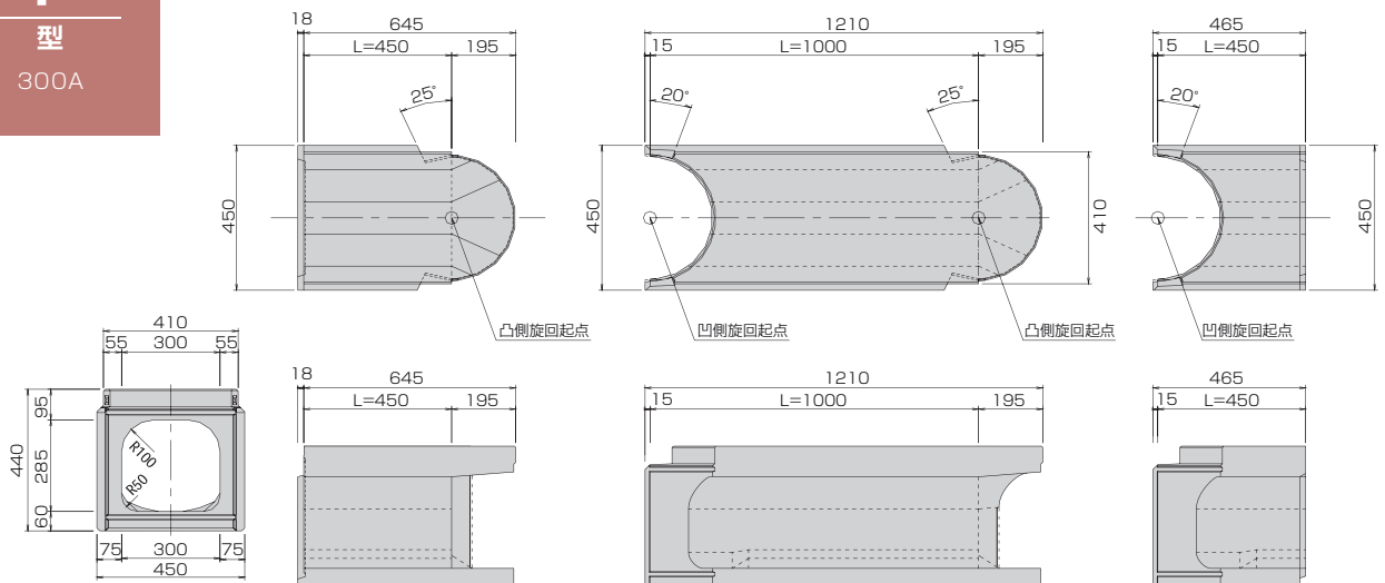
F型300A(凸側)L=450 本体参考重量 150kg
