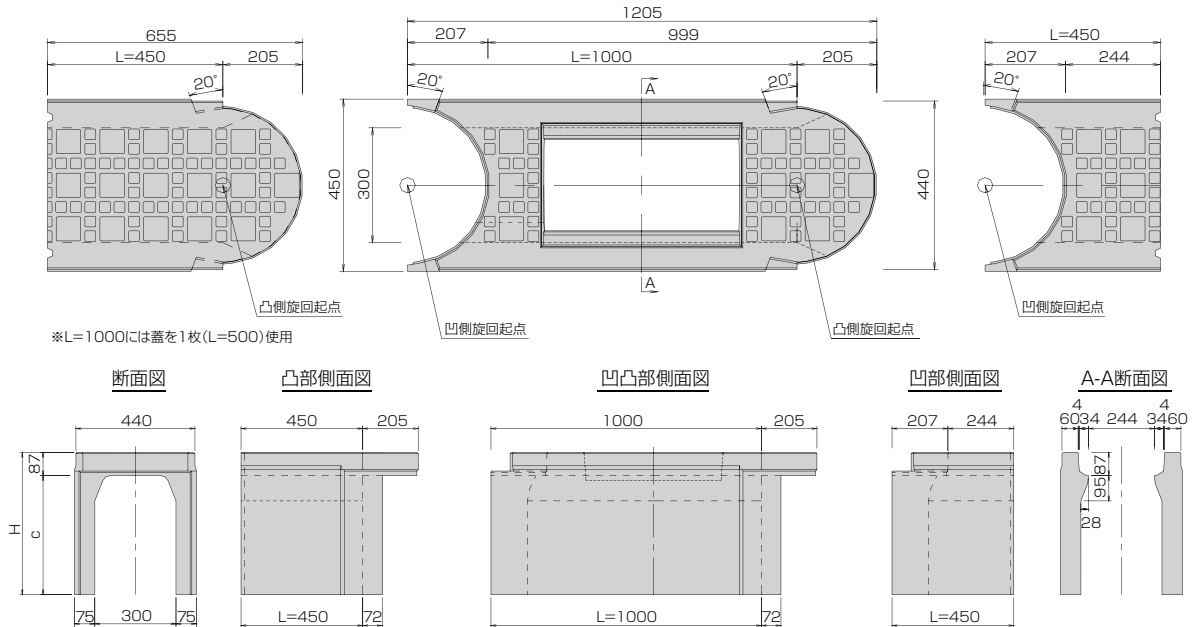
フレキシブルFX可変側溝規格寸法表
